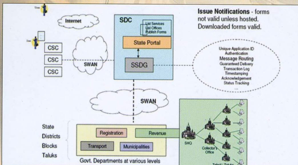
SSDG Wrokflow
